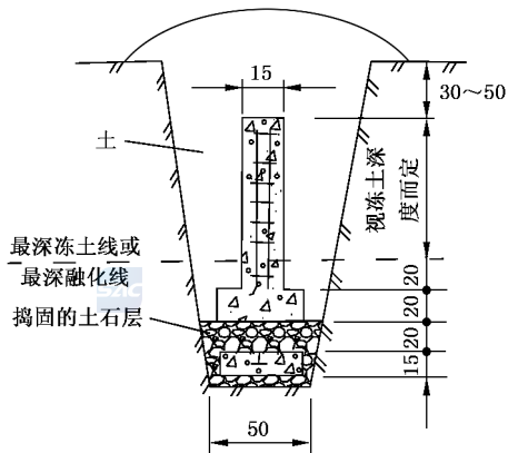
图 B.8 冻土基本标石
