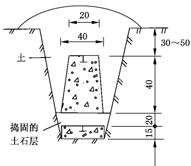
图 B.10 普通标石
