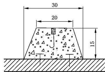
图 B.11 建筑物上标石
