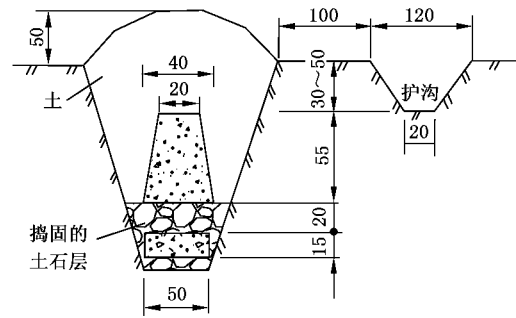
图 B.7 普通基本标石
