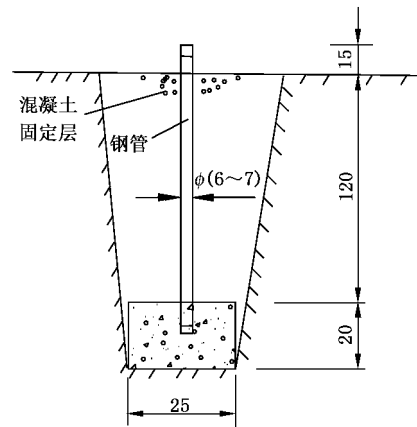
图 B.9 固定沙丘基本标石
