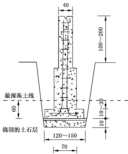
图 B.6 土层天线墩
